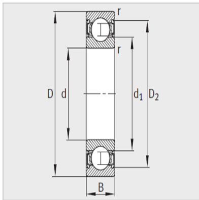
Dichtung 2RSR
